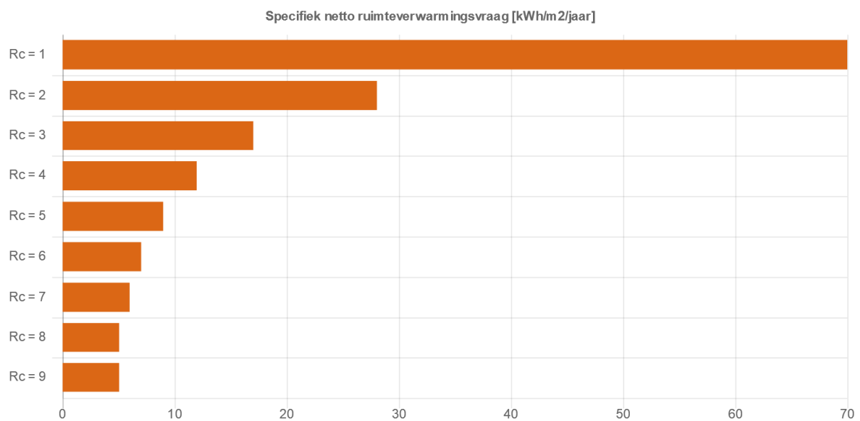
Figuur 14: Netto warmtevraag van een typisch Nederlandse rijtjeswoning met goede kierdichting ( Q_v=0.4 dm 3 /s/m 2 ) en geïsoleerd glas/kozijn ( U=1 W/m 2 /K voor verschillende R_c waarden voor de gesloten geveldelen.
